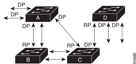
図 18-1 スパンニング ツリー トポロジ
