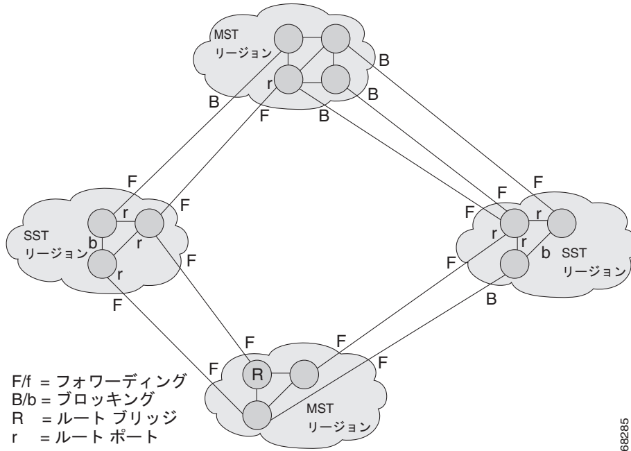
図 18-2 SST および MST リージョンが相互接続されているネットワーク
