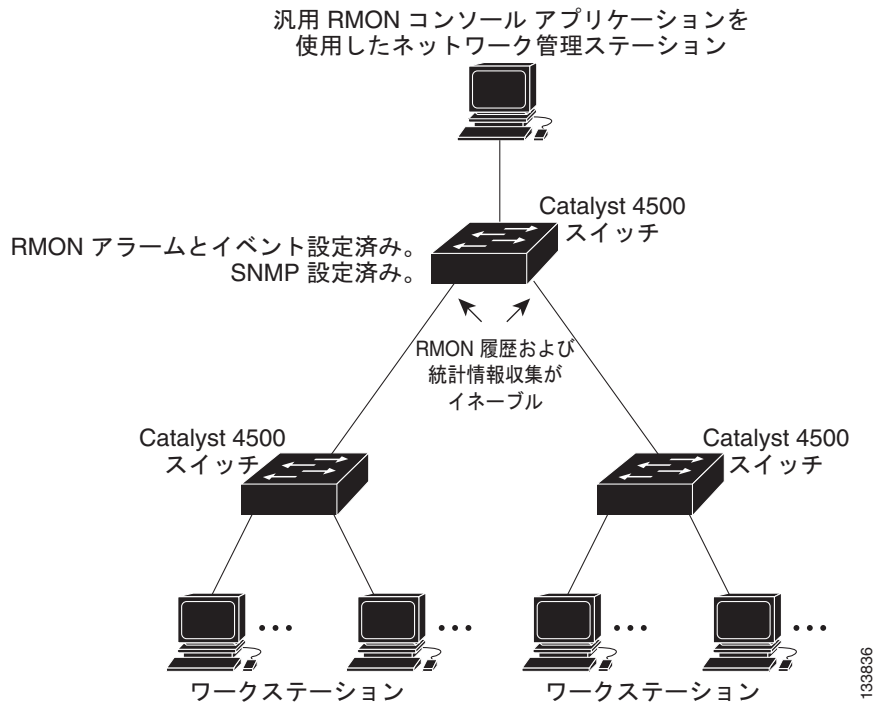
図 58-1 リモート モニタリングの例
