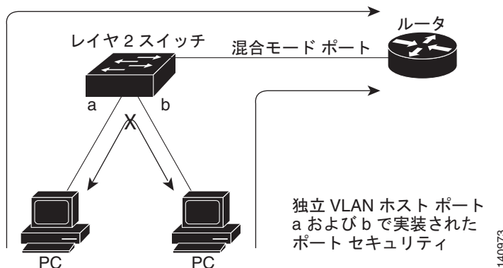
図 43-1 独立 PVLAN ホスト ポートのポートセキュリティ
