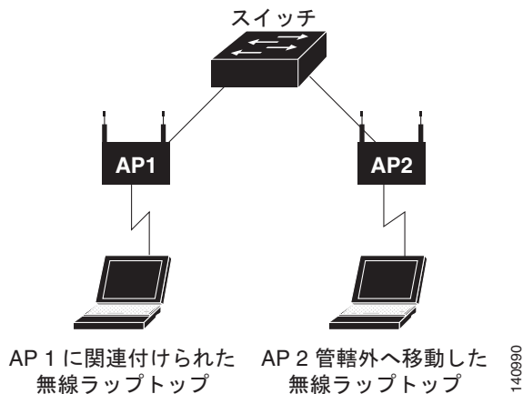
図 43-3 ワイヤレス環境でのポートセキュリティ
