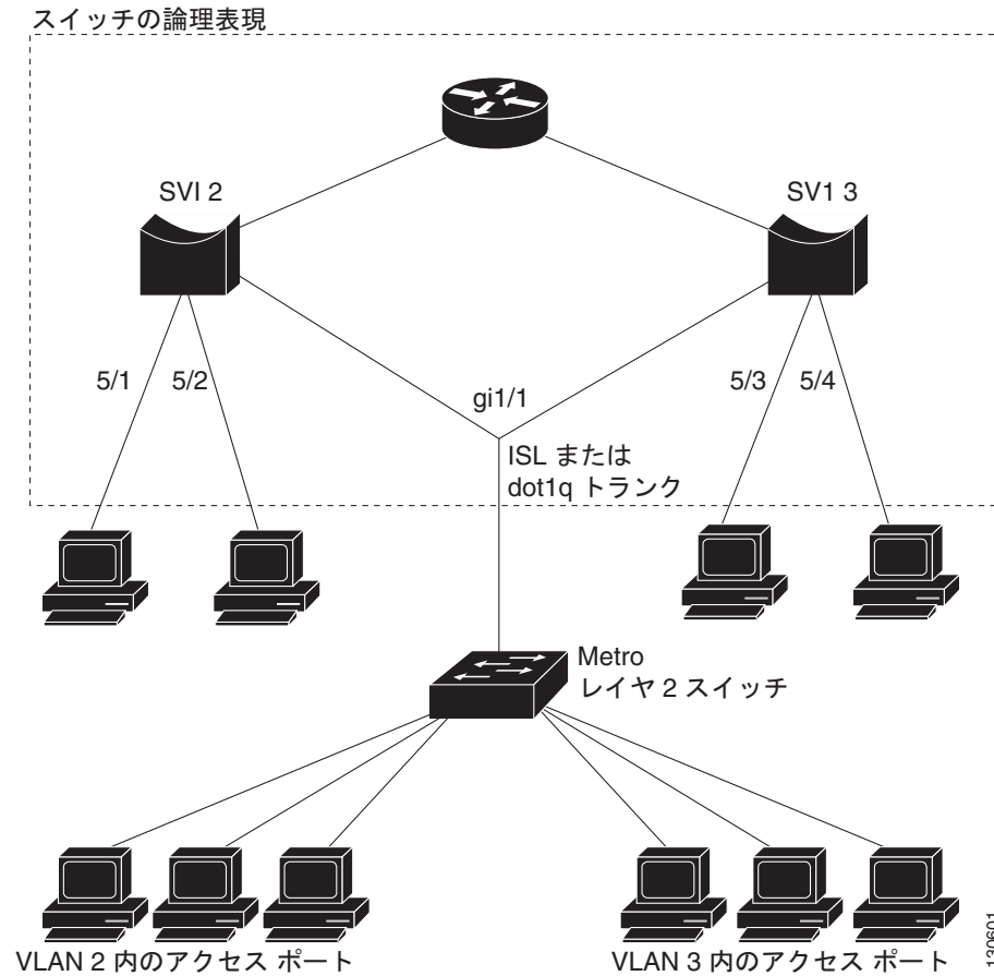
図 43-2 トランク ポートセキュリティ
