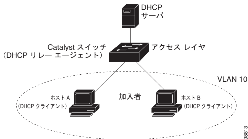
図 45-1 メトロポリタンイーサネットネットワークの DHCP リレー エージェント
