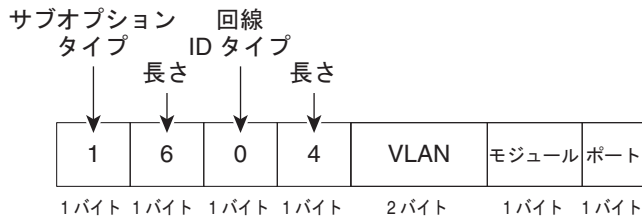
図 45-2 サブオプション packets 形式
