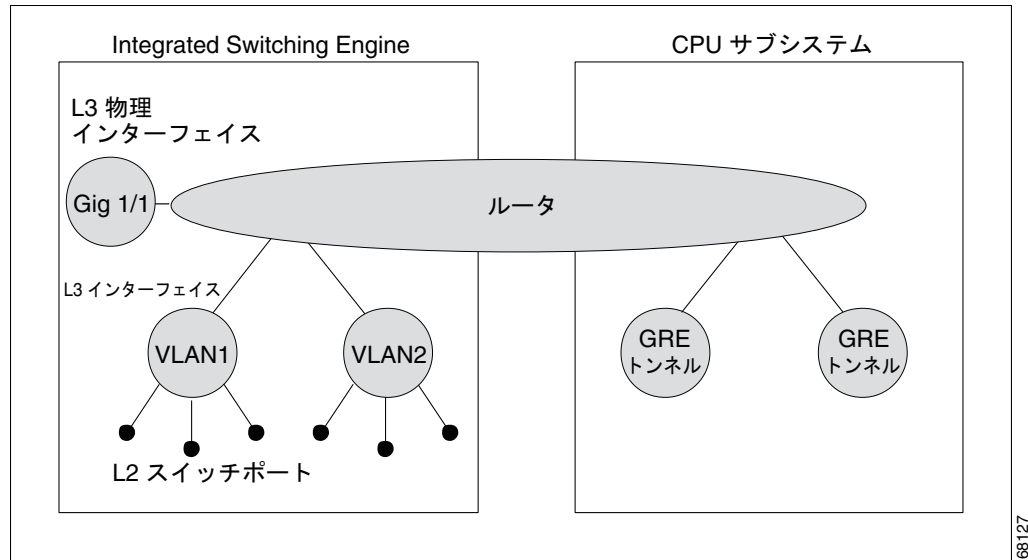
図 31-2 ハードウェアおよびソフトウェア スイッチングのコンポーネント
