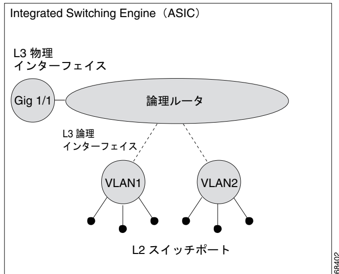
図 31-1 論理 L2/L3 スイッチング コンポーネント
