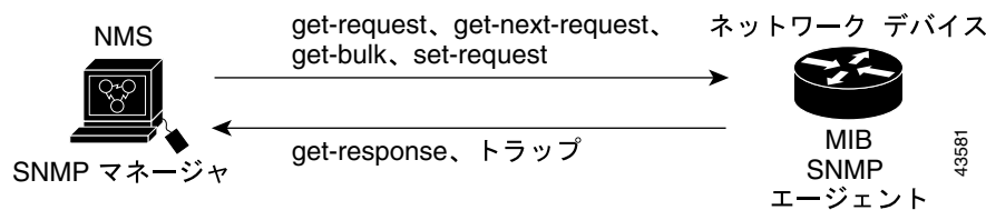
図 48-1 SNMP ネットワーク
