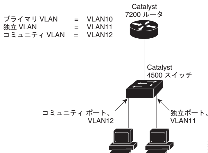
図 37-4 混合モード PVLAN トランク ポート
