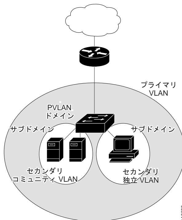
図 37-1 PVLAN のドメイン
