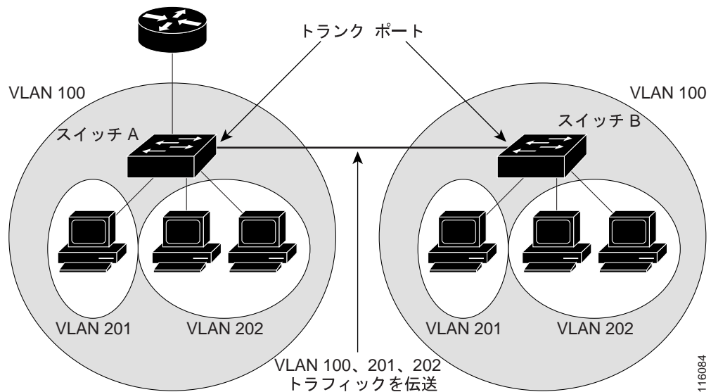
図 37-2 スwitchのプライベート VLAN
