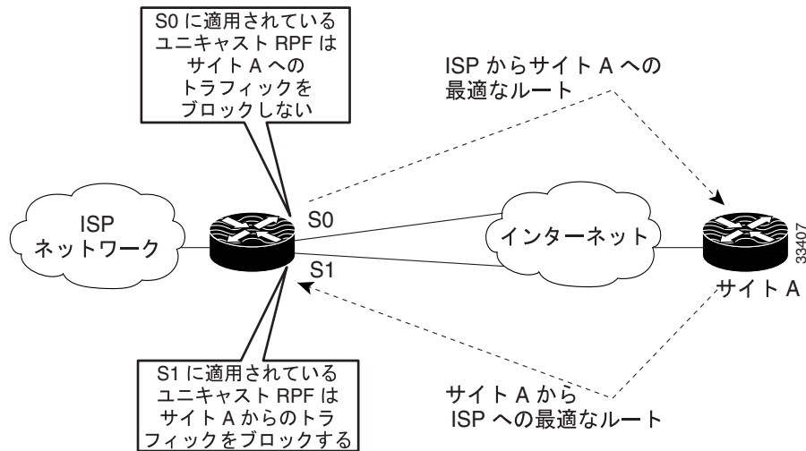
図 31-5 非対称ルーティング環境においてトラフィックをブロックするユニキャスト RPF
