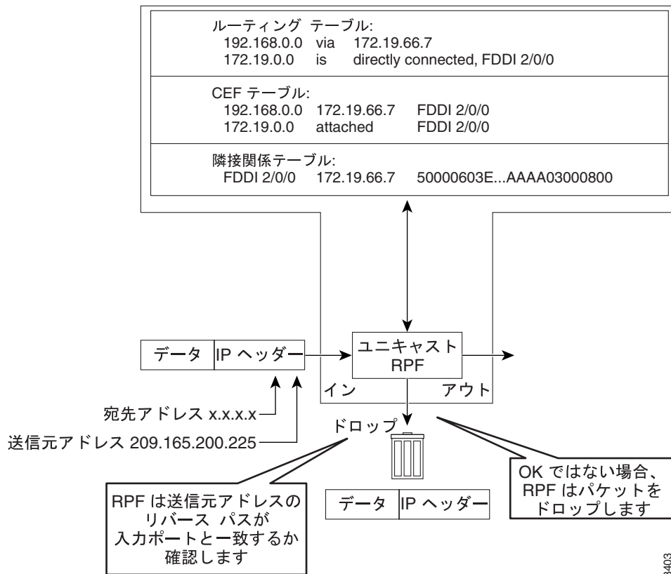
図 31-2 ユニキャスト RPF による確認に失敗したパケットのドロップ
