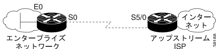
図 31-3 入力フィルタリングのためにユニキャスト RPF を使用するエンタープライズ ネットワーク
