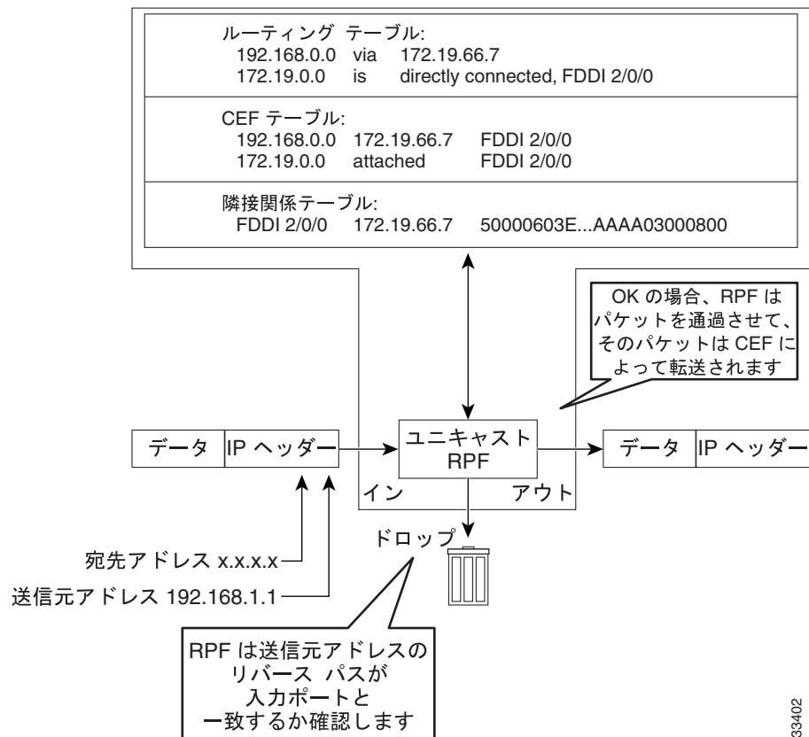
図 31-1 ユニキャスト RPF による IP 送信元アドレスの確認
