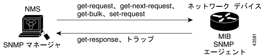
図 47-1 SNMP ネットワーク
