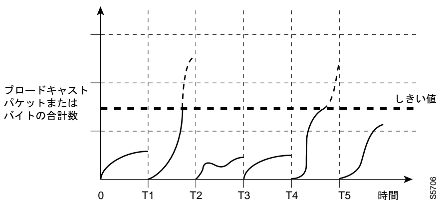
図 44-1 ストーム制御の例 — ハードウェアベースの実装
