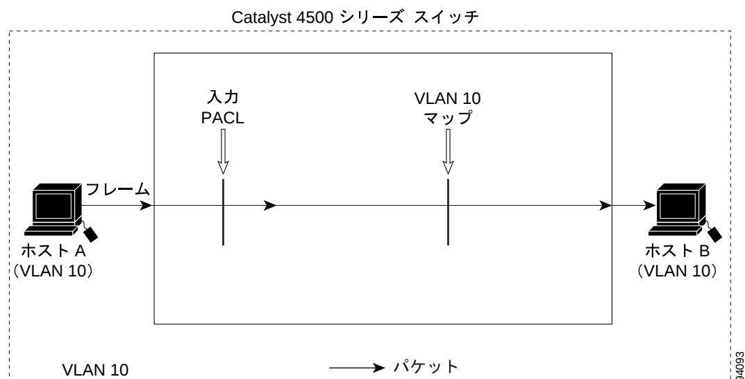
図 42-8 シナリオ 2：VACL との PACL の相互作用
