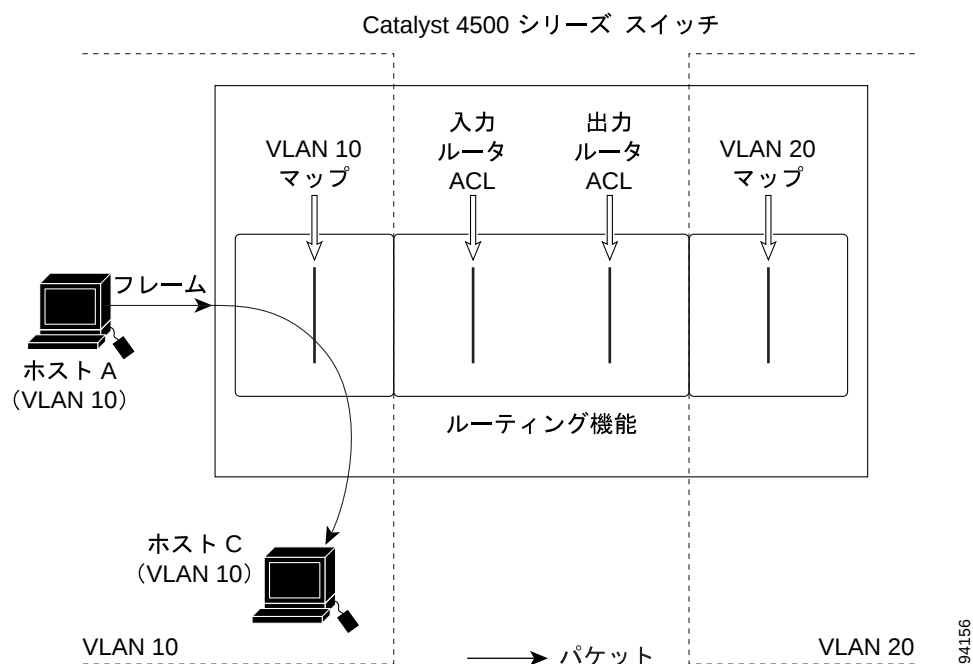
図 42-5 スイッチド パケットへの ACL の適用
