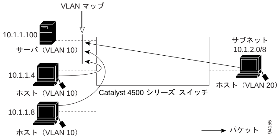
図 42-4 別の VLAN にあるサーバへのアクセスの拒否
