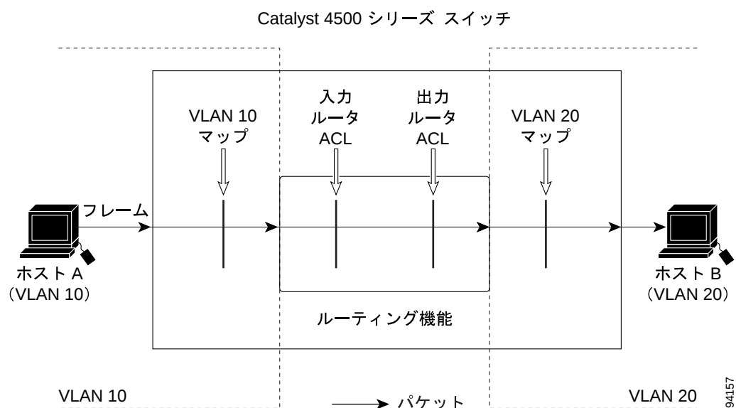
図 42-6 ルーテッド パケットへの ACL の適用
