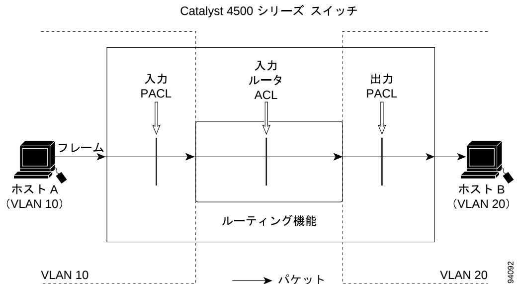
図 42-7 シナリオ 1：入力ルータ ACL との PACL の相互作用
