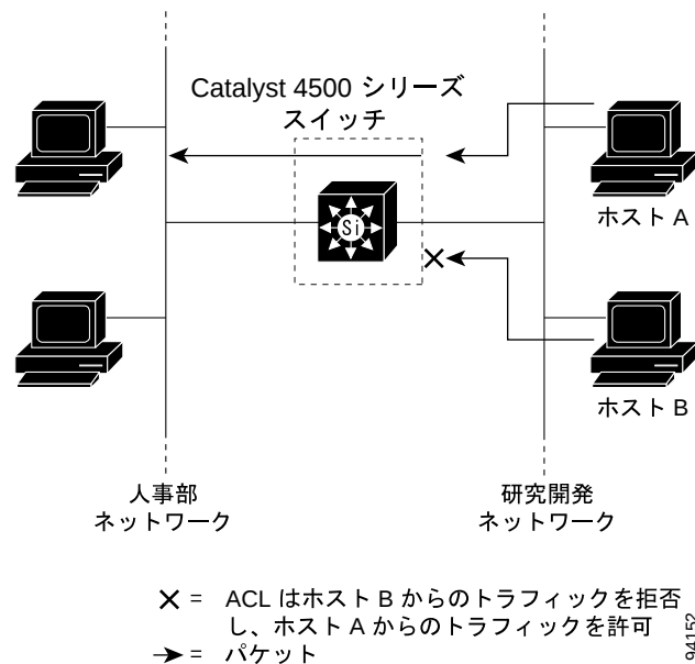
図 42-1 ACL によるネットワーク トラフィックの制御
