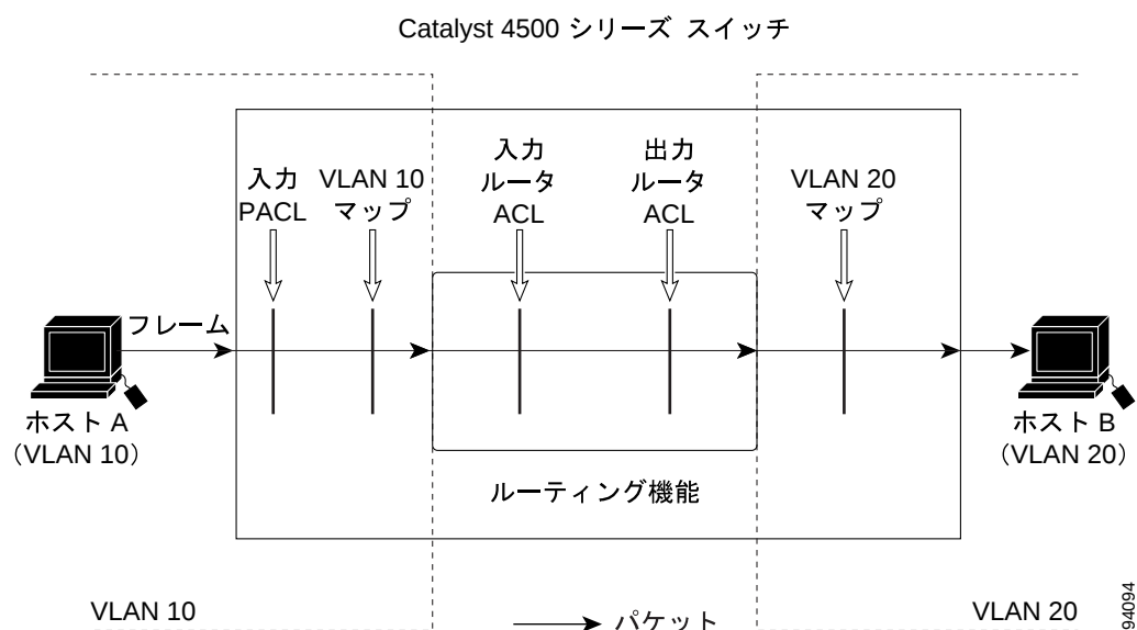
図 42-9 シナリオ 3：VACL と入力ルータ ACL
