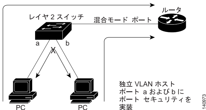
図 38-1 独立 PVLAN ホストポートのポートセキュリティ
