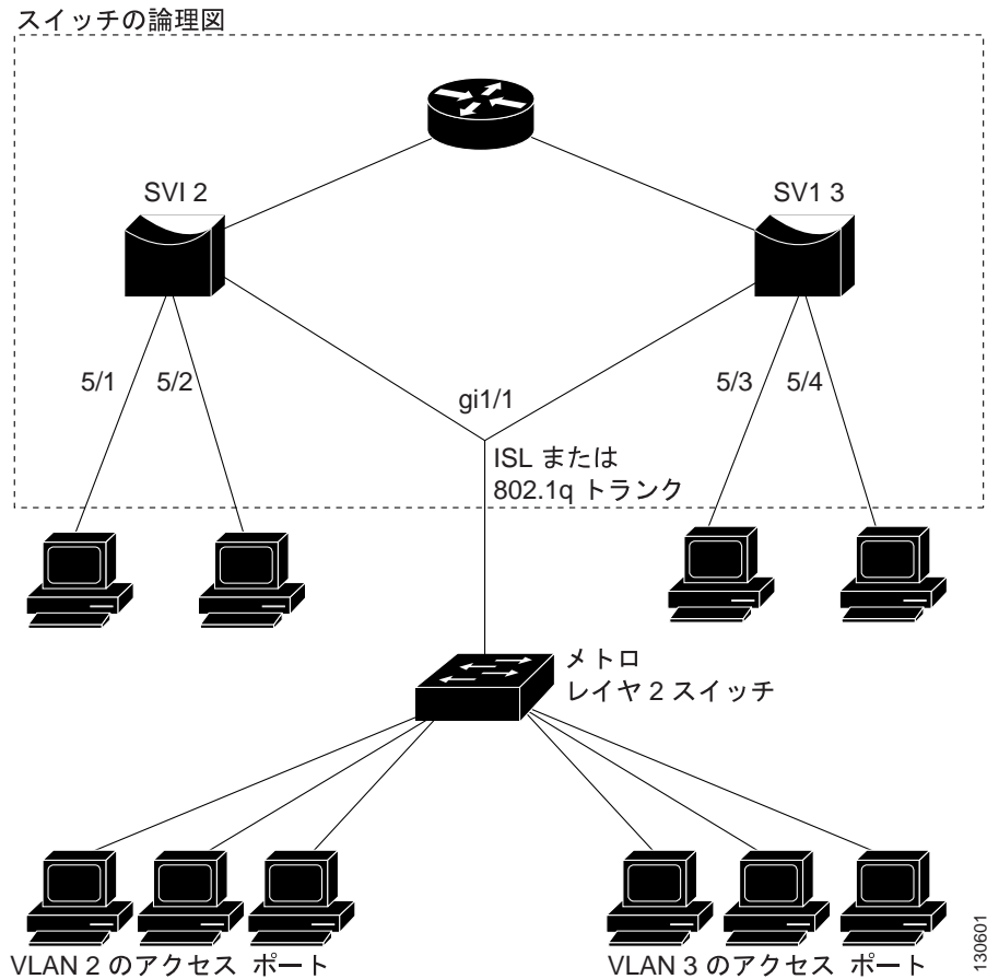
図 38-2 トランク ポート セキュリティ
