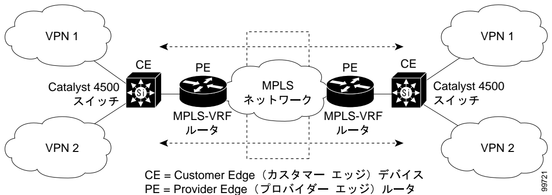
図 33-1 複数の仮想 CE として動作する Catalyst 4500 シリーズ スイッチ
