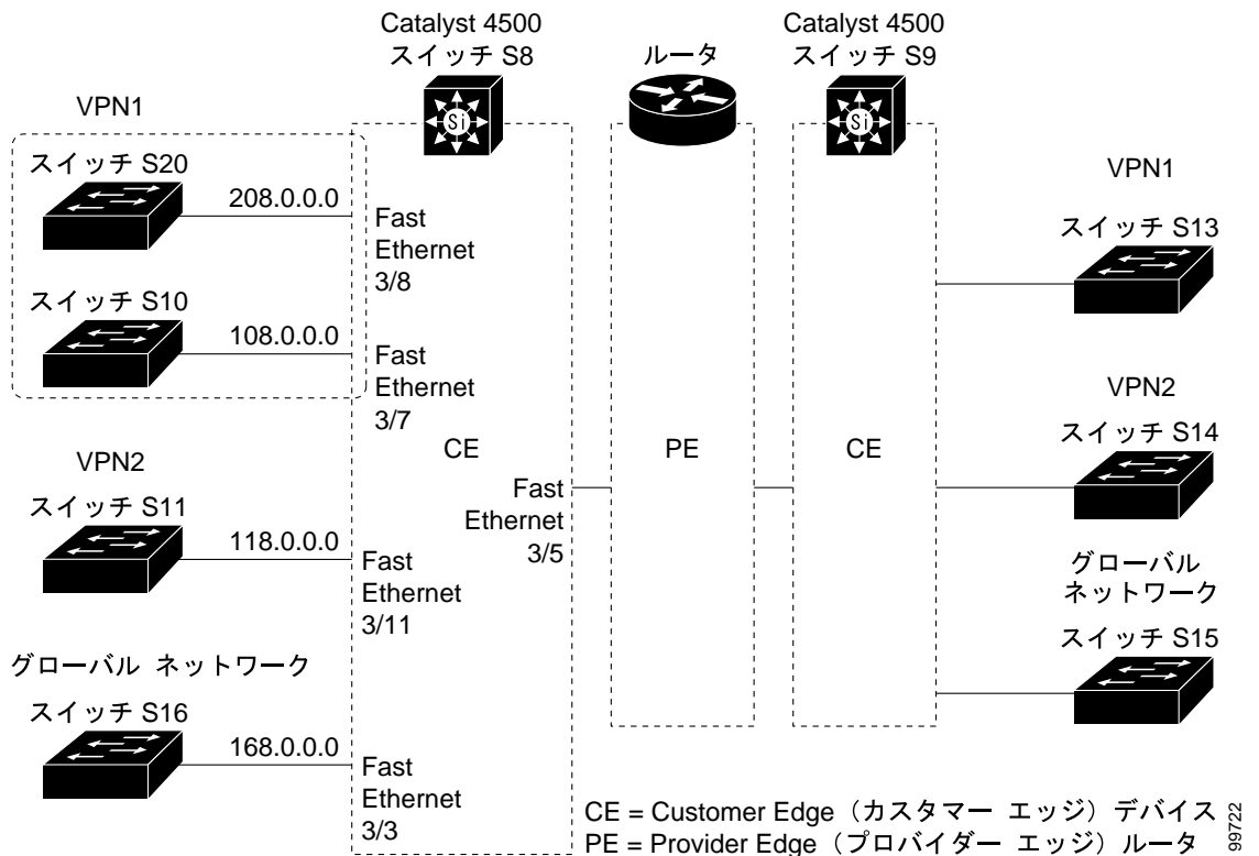
図 33-2 VRF-Lite の設定例
