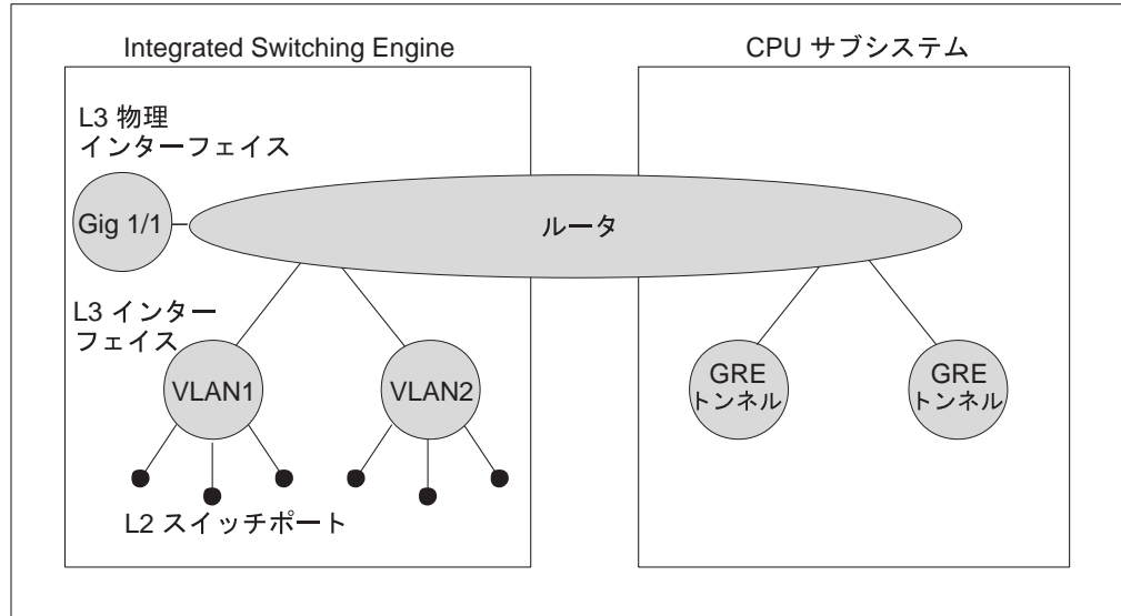
図 28-2 ハードウェアおよびソフトウェア スイッチングのコンポーネント
