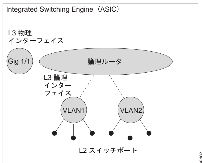
図 28-1 論理 L2/L3 スwitchング コンポーネント
