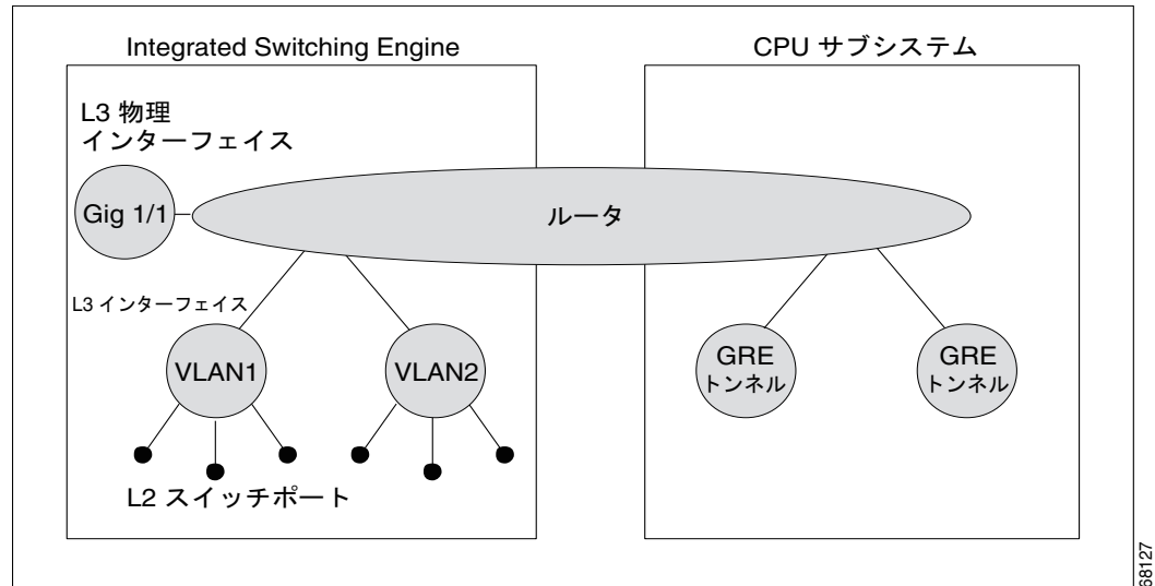
図 26-2 ハードウェアおよびソフトウェア スイッチングのコンポーネント
