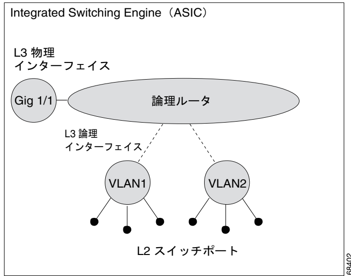
図 26-1 論理 L2/L3 スイッチング コンポーネント
