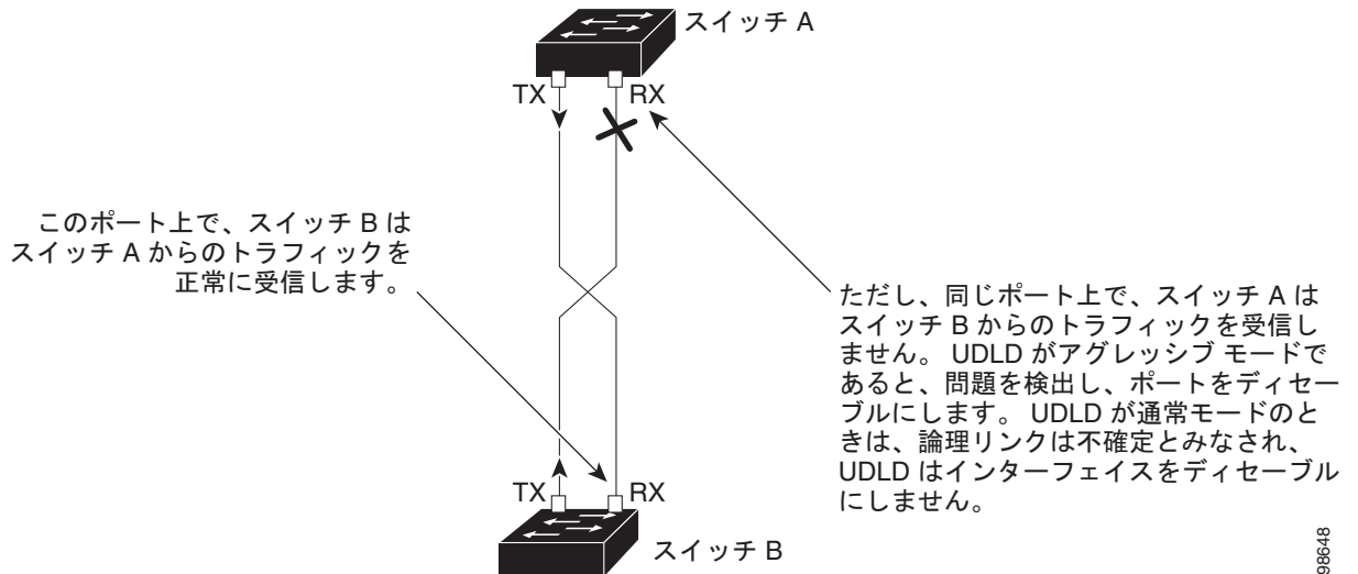
図 28-1 UDLD による単一方向リンクの検出
