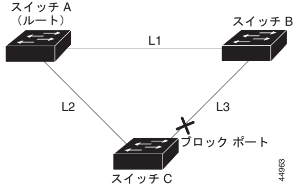
図 20-6 間接リンク障害発生前の BackboneFast の例
