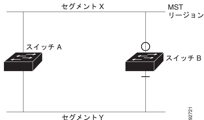
図 19-2 標準スイッチおよび先行標準のスイッチでの相互運用
