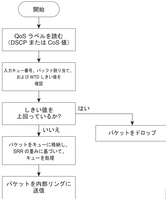
図 34-8 入力ポートのキューイングおよびスケジューリング フローチャート
