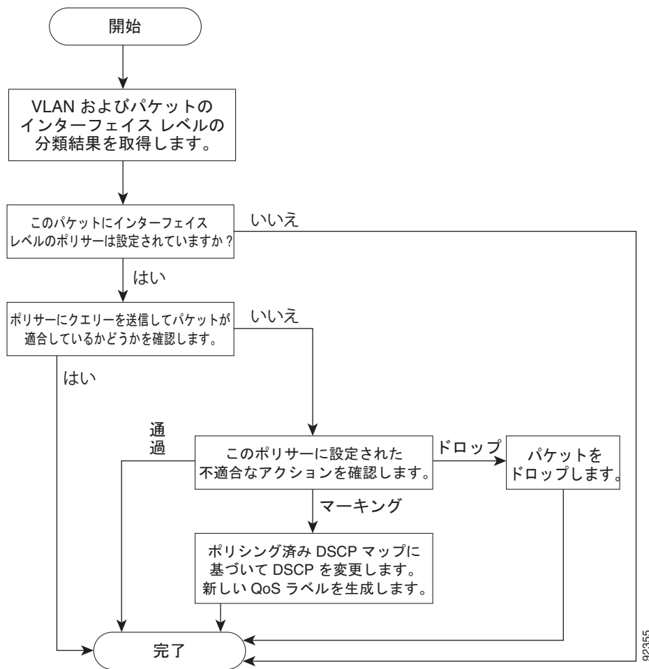
図 34-5 SVI のポリシー マップおよびマーキング フローチャート
