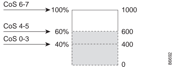
図 34-7 WTD およびキューの動作
