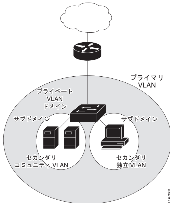
図 16-1 プライベート VLAN ドメイン
