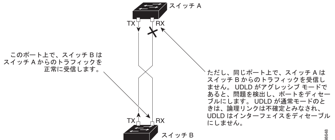
図 28-1 UDLD による単一方向リンクの検出
