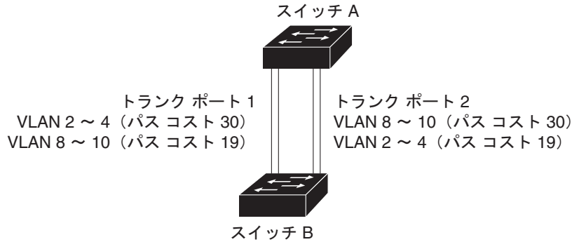
図 14-4 パス コストによってトラフィックが分散される負荷分散トランク
