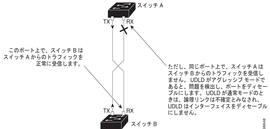
図 29-1 UDLD による単一方向リンクの検出
