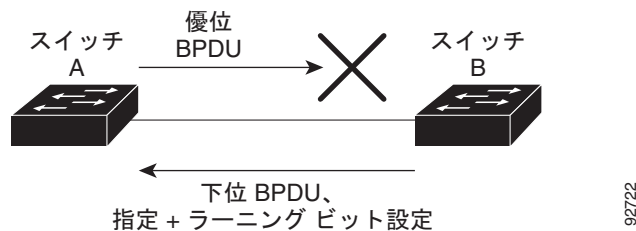
図 20-3 単一方向リンクの失敗の検出
