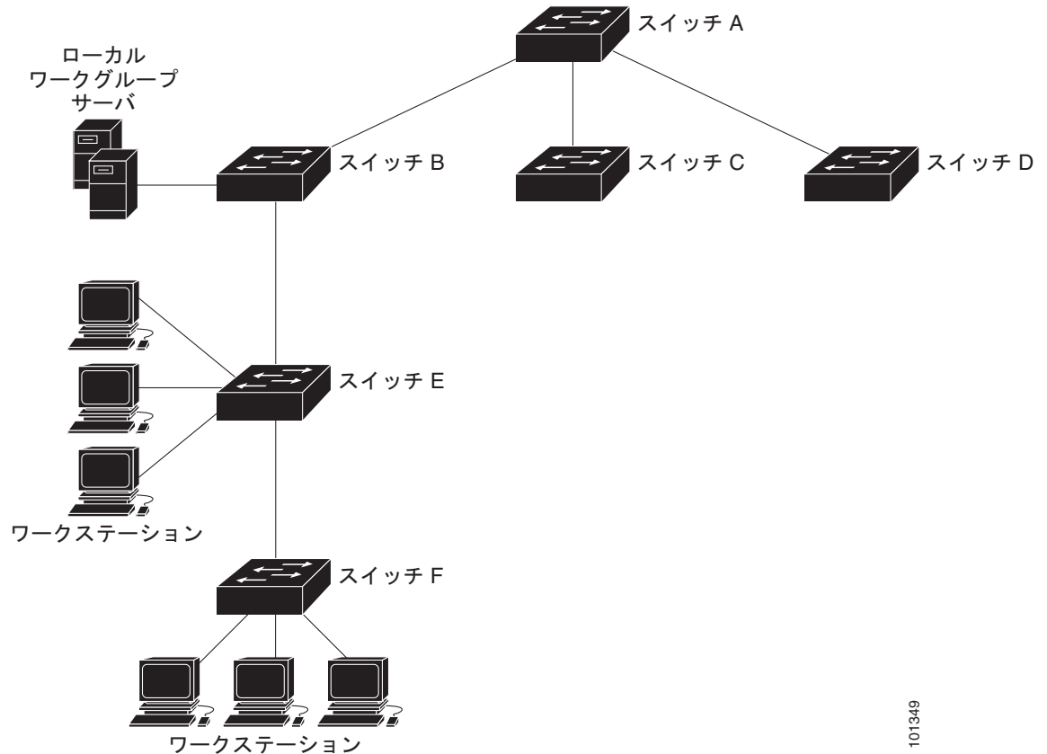
図 8-1 一般的な NTP ネットワークの構成
