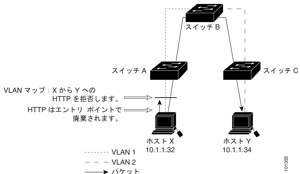
図 32-4 配線クローゼットの構成
