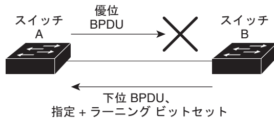
図 22-3 単一方向リンクの失敗の検出
