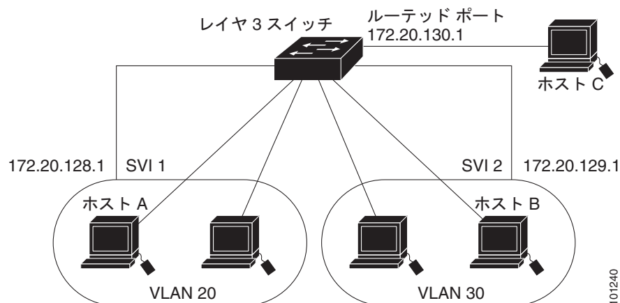
図 54-1 フォールバックブリッジネットワークの例
