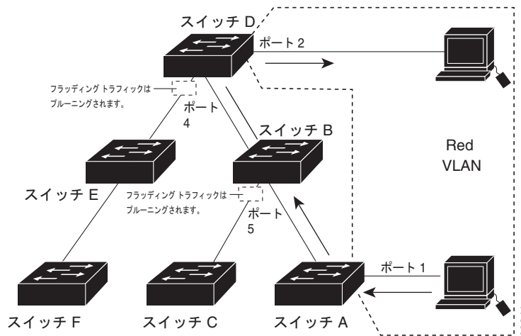
図 16-2 VTP プルーニングによるフラッディング ट्रフィックの最適化
