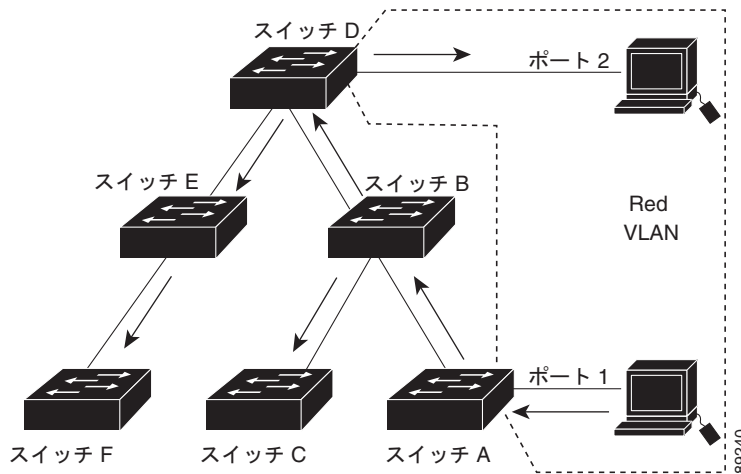
図 16-1 VTP プルーニングを使用しない場合のフラッディング ट्रフィック
