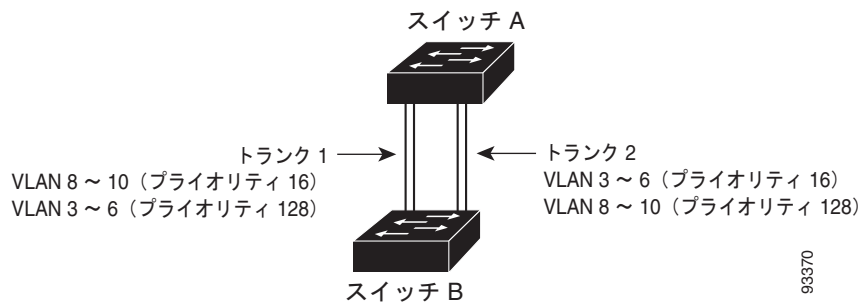
図 15-3 STP ポート プライオリティによる負荷分散
