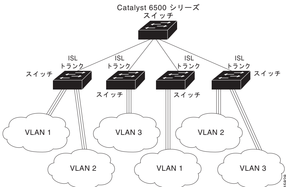
図 15-2 ISL トランキング環境のスイッチ
