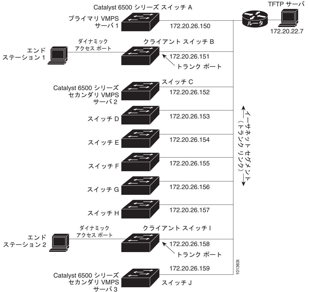
図 15-5 ダイナミック ポート VLAN メンバシップの構成例
