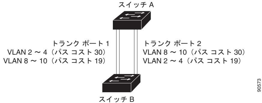
図 15-4 パス コストによってトラフィックが分散される負荷分散トランク
