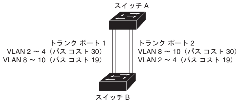
図 15-1 論理的に定義されたネットワークとしての VLAN
