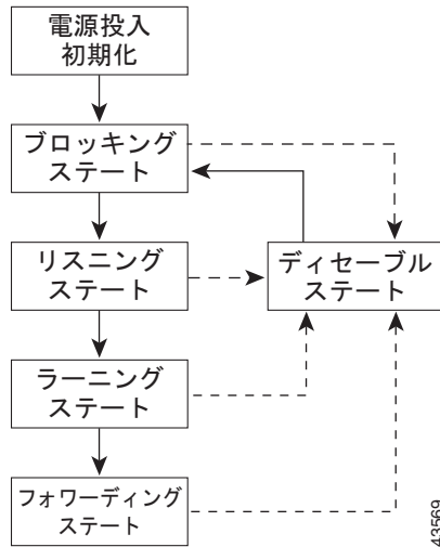
図 20-2 スパニング ツリー インターフェイス ステート
