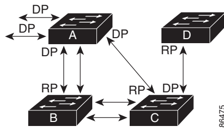
図 20-3 スパンニング ツリー トポロジ
