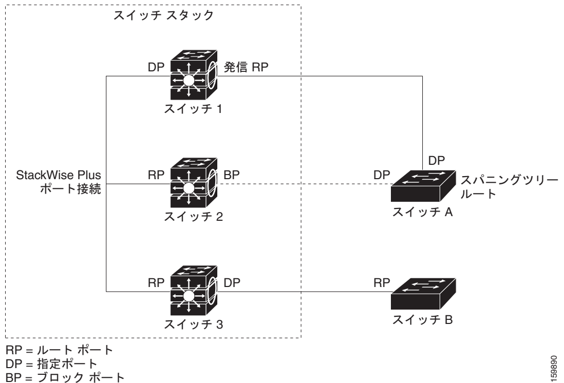
図 20-1 スイッチ スタックでのスパニング ツリー ポート ステート
