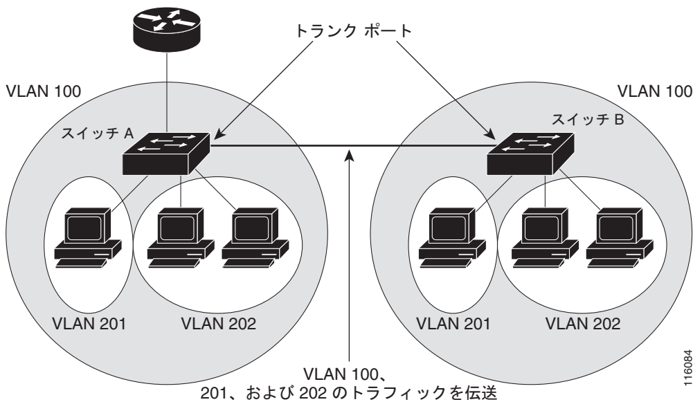
図 18-2 複数のスイッチにまたがるプライベート VLAN
