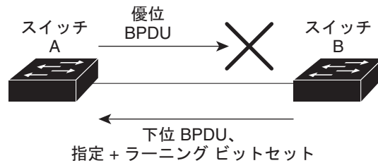
図 21-3 単一方向リンクの失敗の検出
