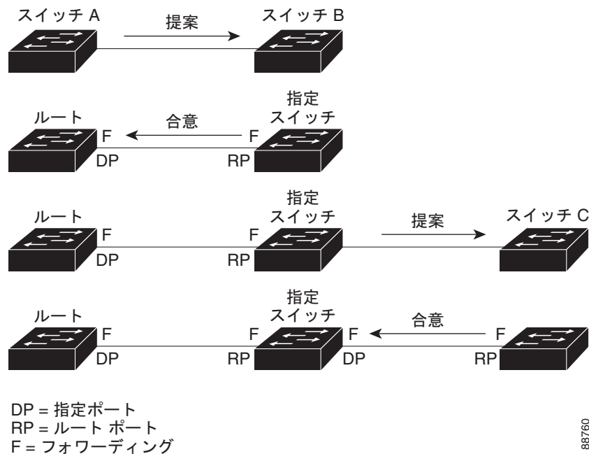
図 21-4 高速コンバージェンスの提案と合意のハンドシェイク
