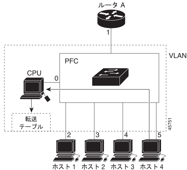
図 26-2 2 番めのホストのマルチキャスト グループへの加入
