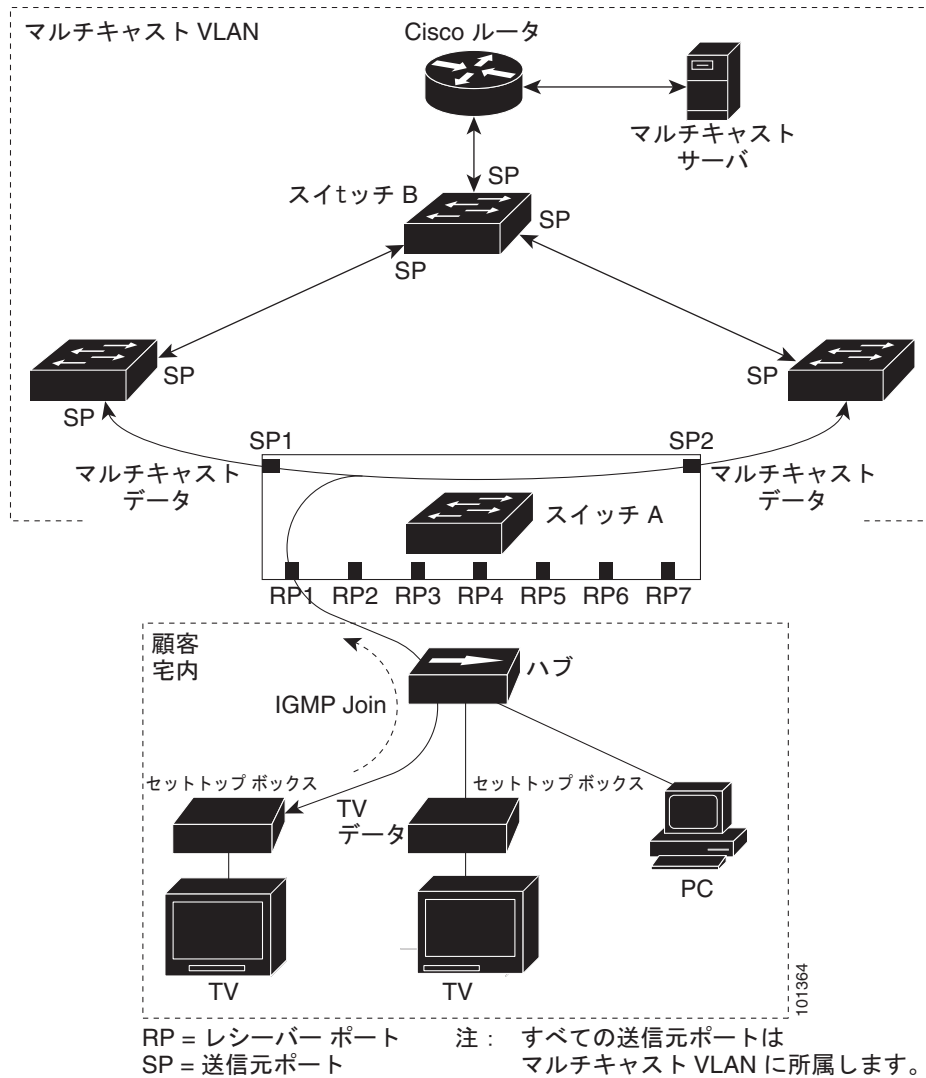
図 26-3 MVR の例
