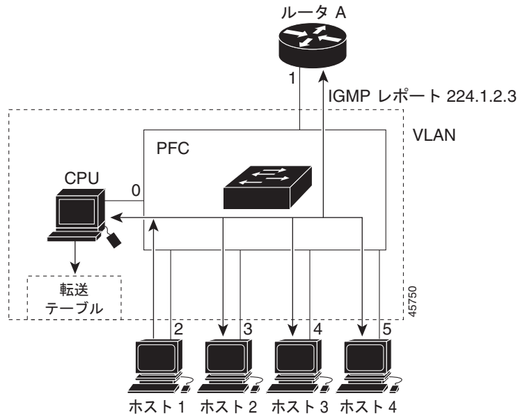
図 26-1 最初の IGMP Join メッセージ
