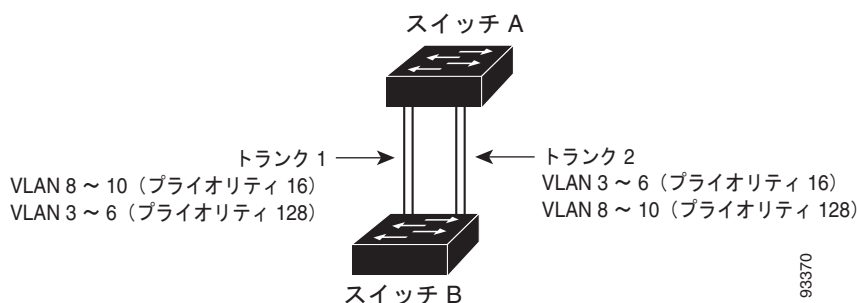
図 14-3 STP ポート プライオリティによるロード シェアリング
