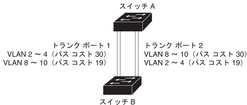
図 14-4 パス コストによってトラフィックが分散されるロード シェアリング トランク
