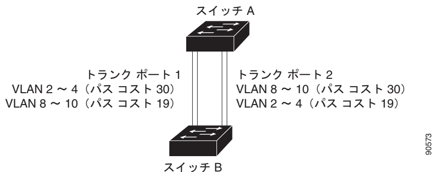
図 14-1 論理的に定義されたネットワークとしての VLAN
