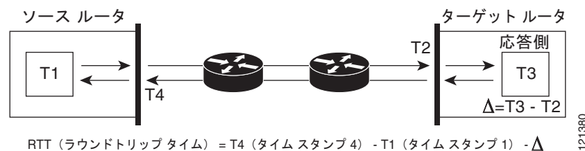
図 44-2 Cisco IOS IP SLA 応答側タイムスタンプ
