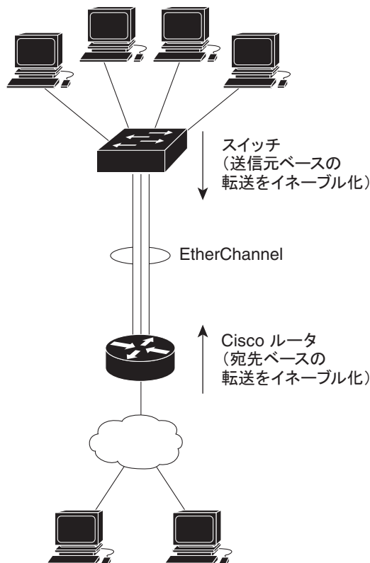
図 39-5 負荷の分散および転送方式
