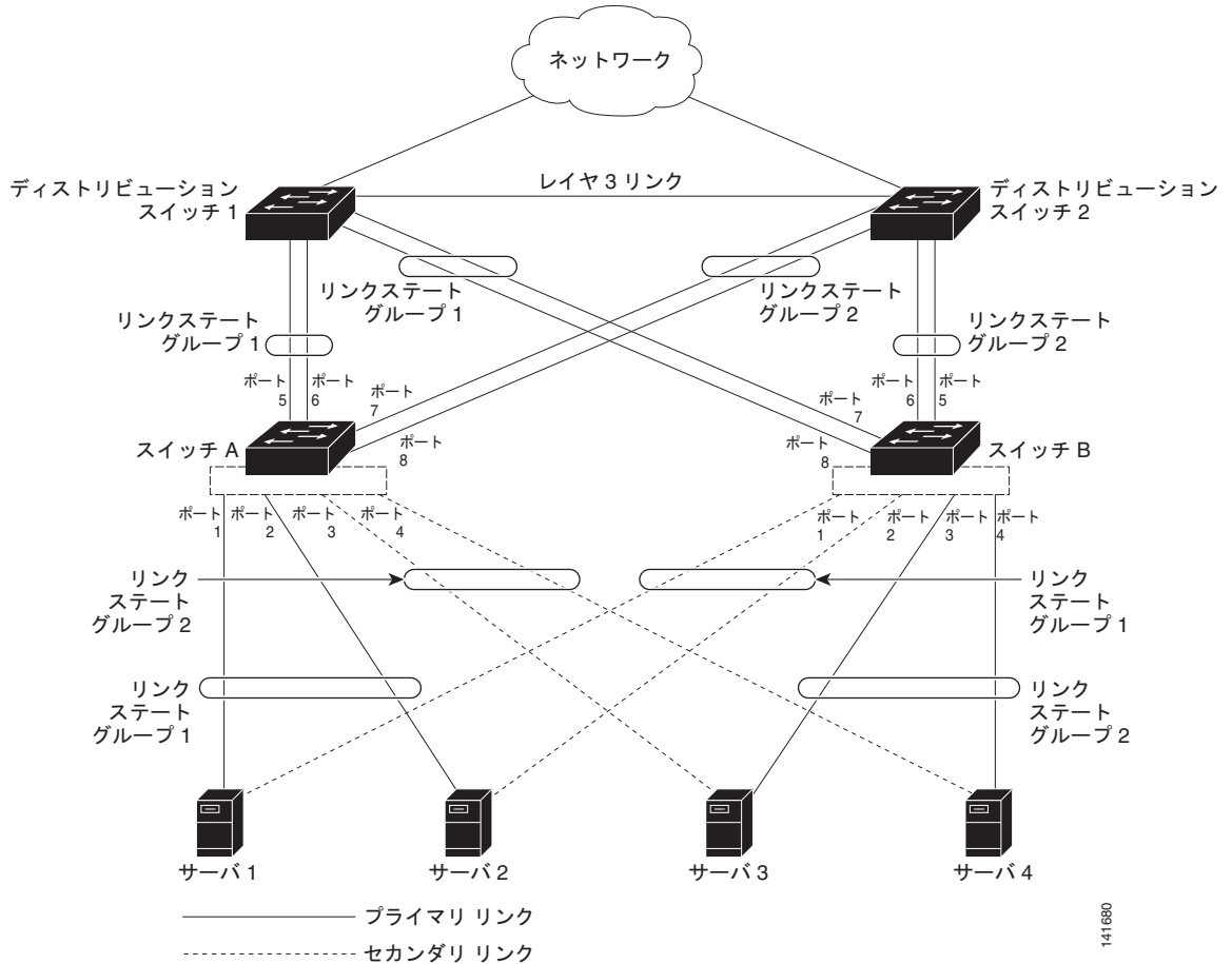
図 39-6 一般的なリンクステートトラッキングの設定
