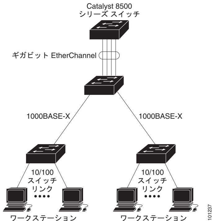
図 39-1 一般的な EtherChannel 構成
