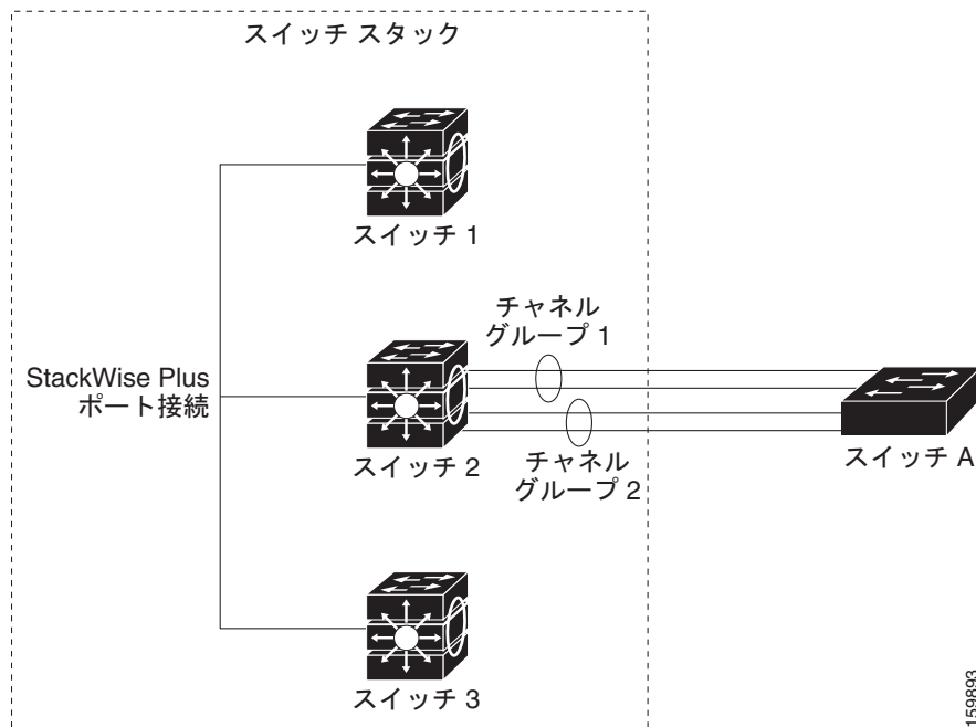
図 39-2 単一スイッチ EtherChannel
