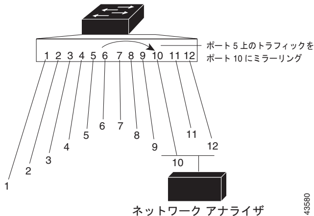
図 32-1 単一スイッチでのローカル SPAN の設定例
