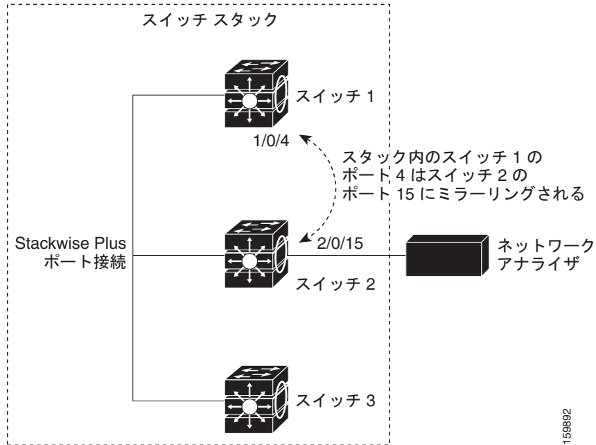
図 32-2 スイッチ スタックでのローカル SPAN の設定例
