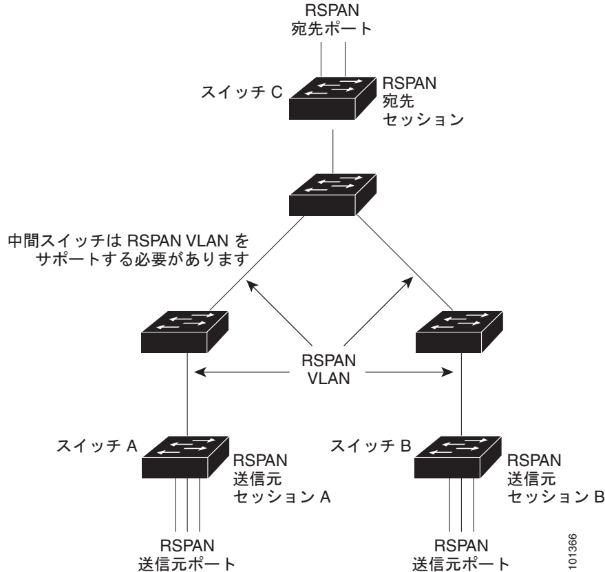
図 32-3 RSPAN の設定例
