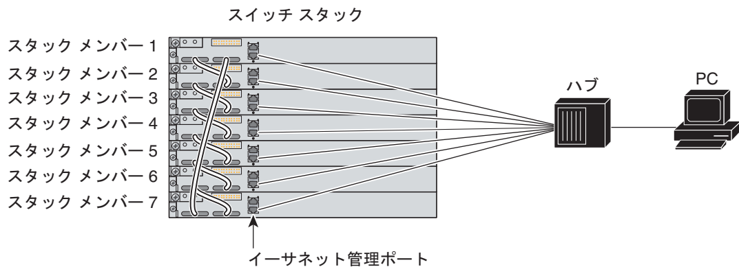
図 12-3 PC とスイッチ スタックの接続
