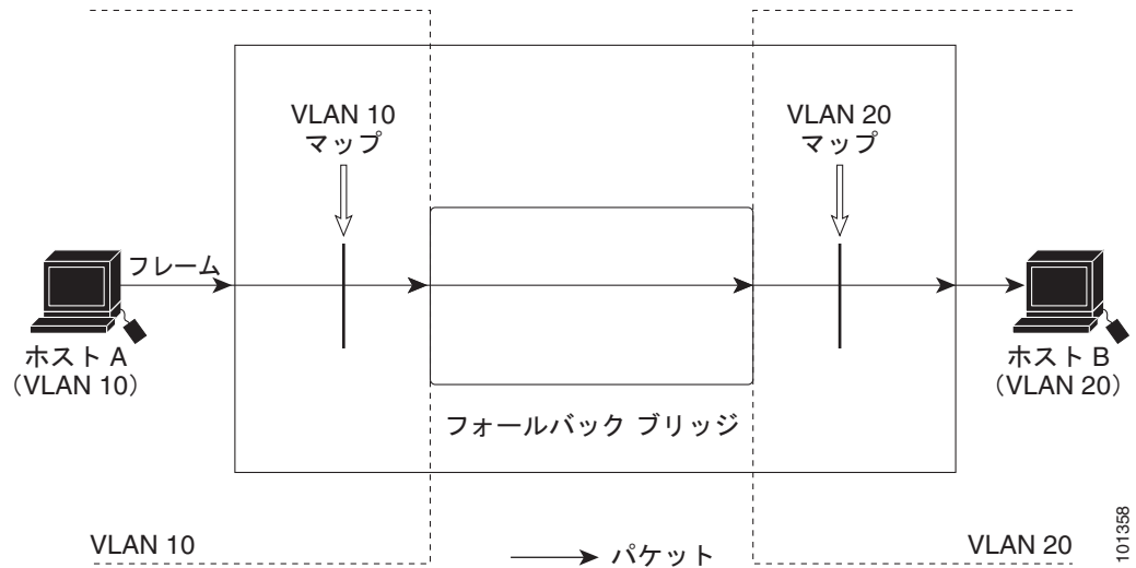
図 35-7 ブリッジド packets への ACL の適用
