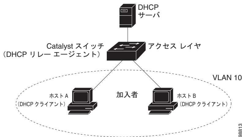
図 21-1 メトロポリタンイーサネット ネットワークにおける DHCP リレー エージェント
