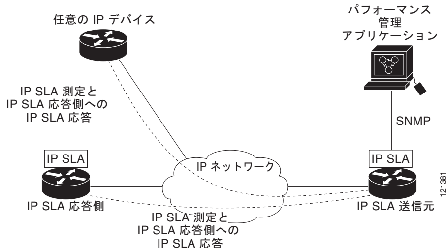
図 44-1 Cisco IOS IP SLA 動作
