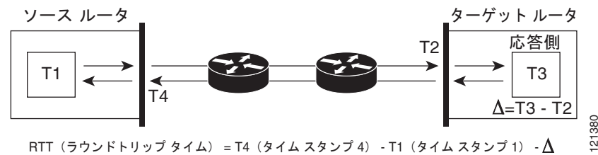
図 44-2 Cisco IOS IP SLA Responder タイム スタンプ
