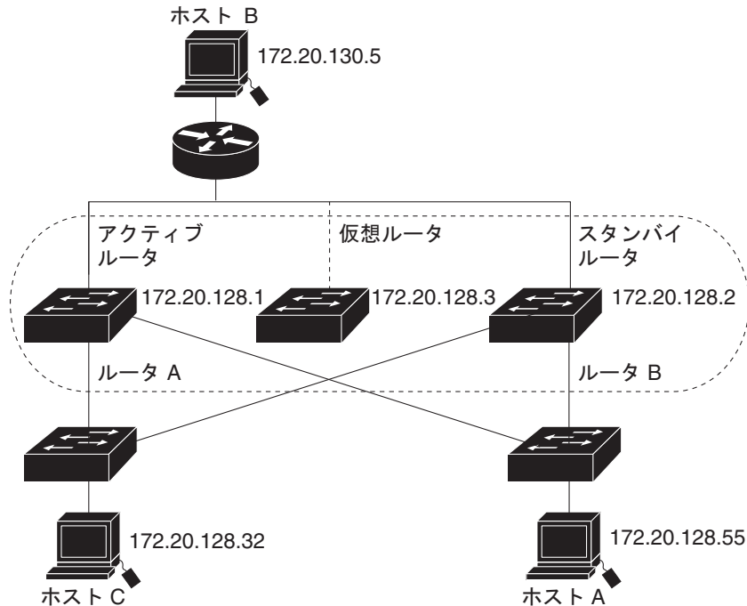
図 43-1 HSRP の一般的な構成
