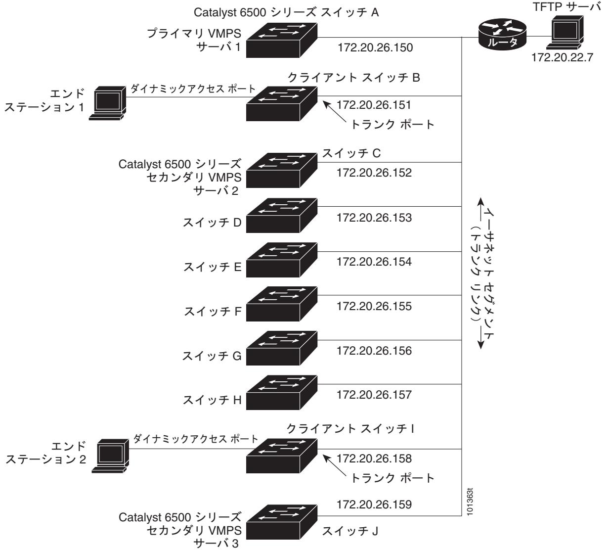
図 13-4 ダイナミック ポート VLAN メンバーシップの構成例
