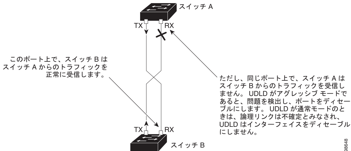
図 27-1 UDLD による単一方向リンクの検出
