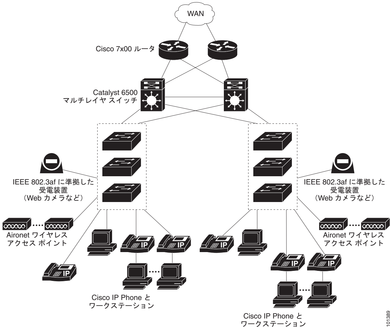
図 1-4 バックボーン構成でのワイヤリング クローゼットのスイッチ
