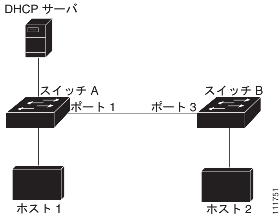
図 21-2 ダイナミック ARP インспекションのためにイネーブルにされた VLAN 上の ARP パケット検証
