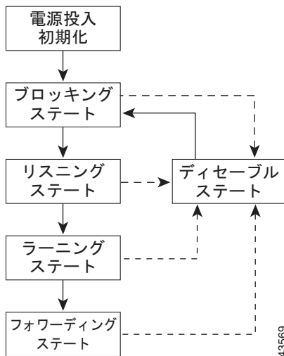
図 26-1 スパンニング ツリー インターフェイス ステート
