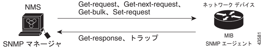
図 31-1 SNMP ネットワーク
