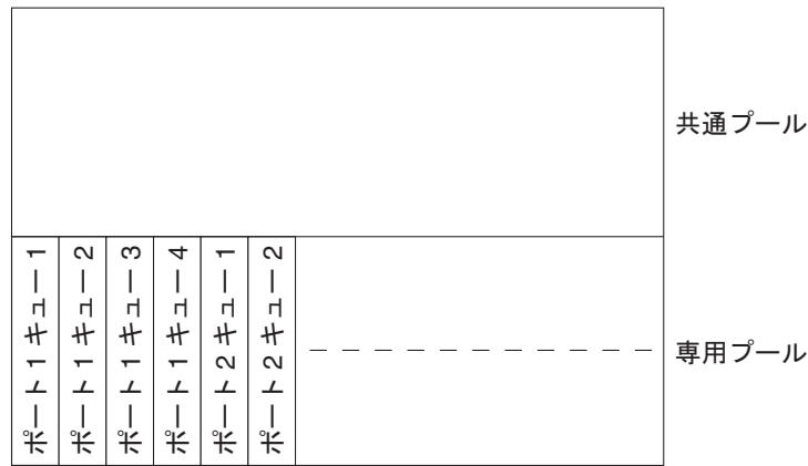
図 34-10 出力キューのバッファ割り当て
