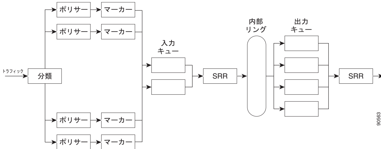
図 34-6 入力および出力キューの位置
