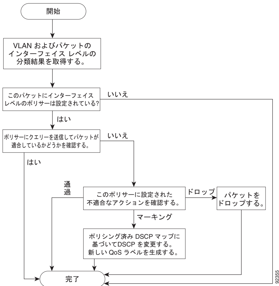
図 34-5 SVI のポリシングおよびマーキング フローチャート
