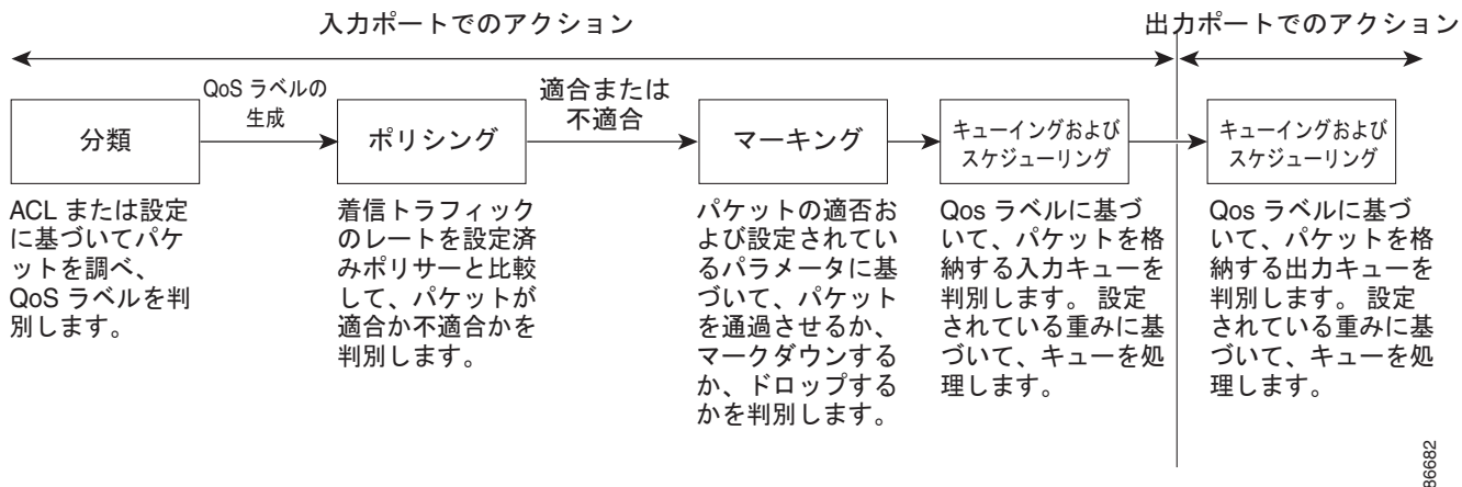
図 34-2 QoS の基本モデル
